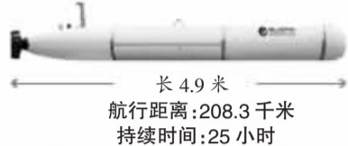
“金枪鱼” 自动水下航行器
