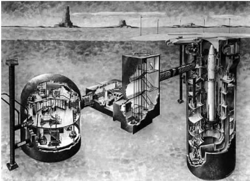
地下导弹发射井示意图:从左到右分别是控制室、连接坑道和导弹竖井。
